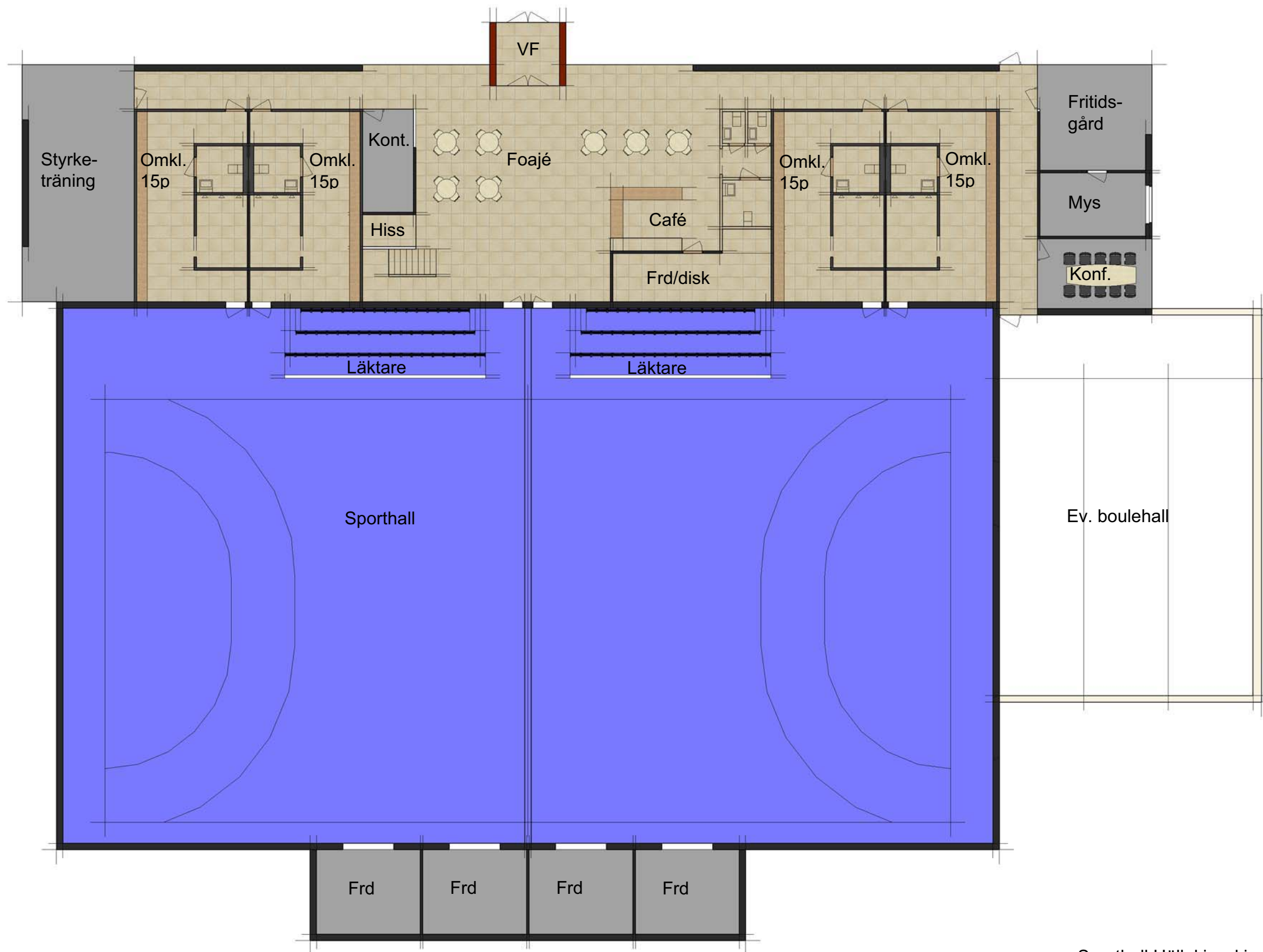
Sporthall Hällekis, skiss 2011.03.01 plan 1:200 [A3] alt B
